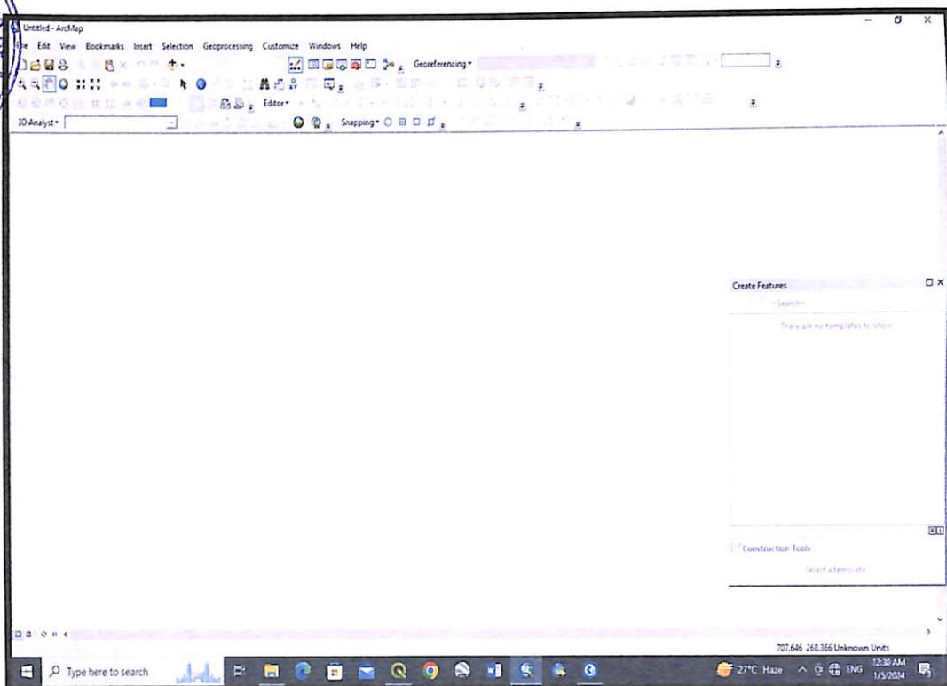
Arc GIS
