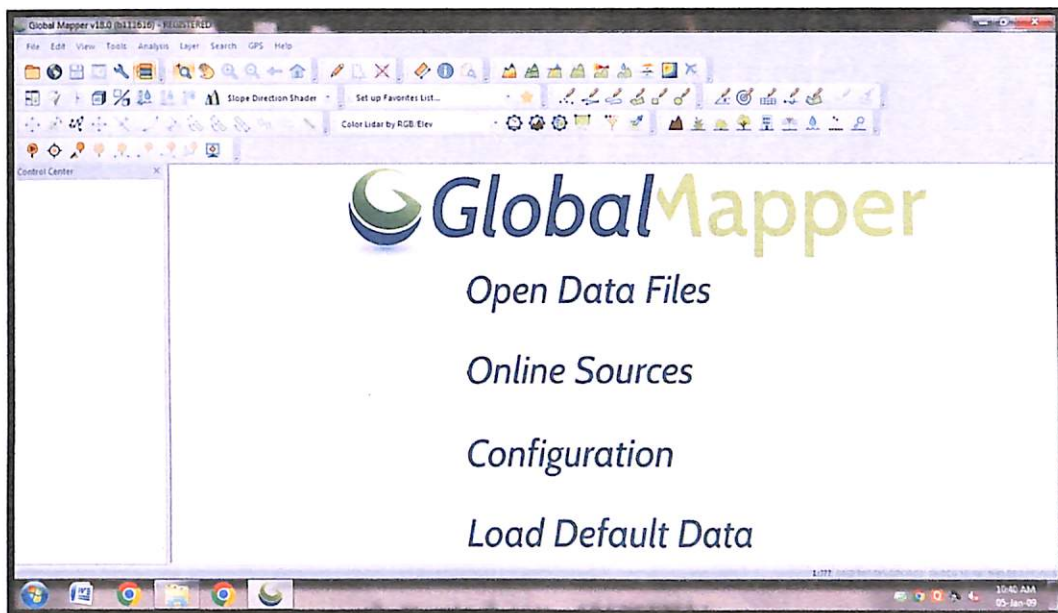
Global Mapper
